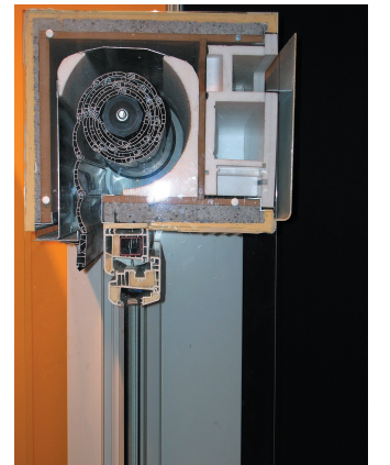
esempio di isolamento del cassonetto
